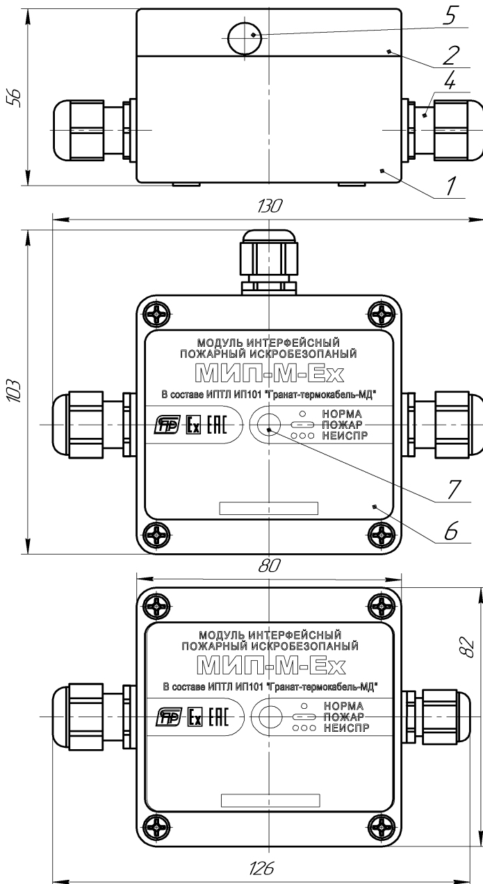
Рис. А.1. Внешний вид модулей МИП-М(-Ех).
