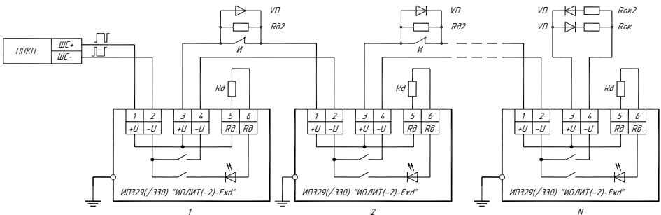
Схема подключения ИП329 «ИОЛИТ-Exd» в двухпроводный дупольярный шлейф сигнализации
