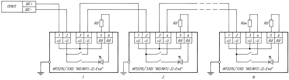
Схема подключения ИП329 «ИОЛИТ-Exd» в двухпроводный однополярный шлейф сигнализации
